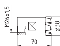
11: Vykrúžovací vrták ø38
