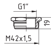
12: Redukce G1"/M42x1,5
