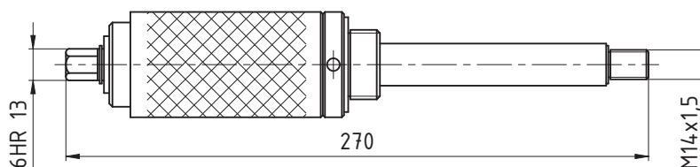
15: Navrtávač
