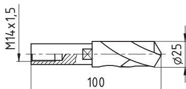
7: Vrták ø24
