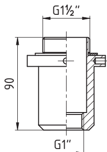
2: Nástavec G1"/G1½"
