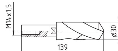
8: Vrták ø30
