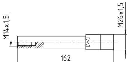
6: Prodloužení M14x1,5/M26x1,5
