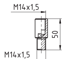
14: Prodloužení M14x1,5/M14x1,5
