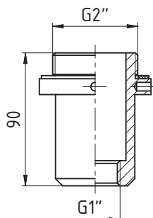
1: Nástavec G1"/G2"
