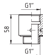
5: Nástavec G1"/G1"
