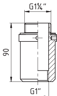
3: Nástavec G1"/G1¼"
