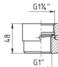
4: Nástavec G1"/G1¼"
