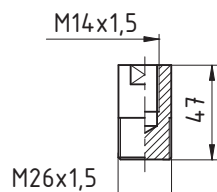
13: Prodloužení M14x1,5/M26x1,5
